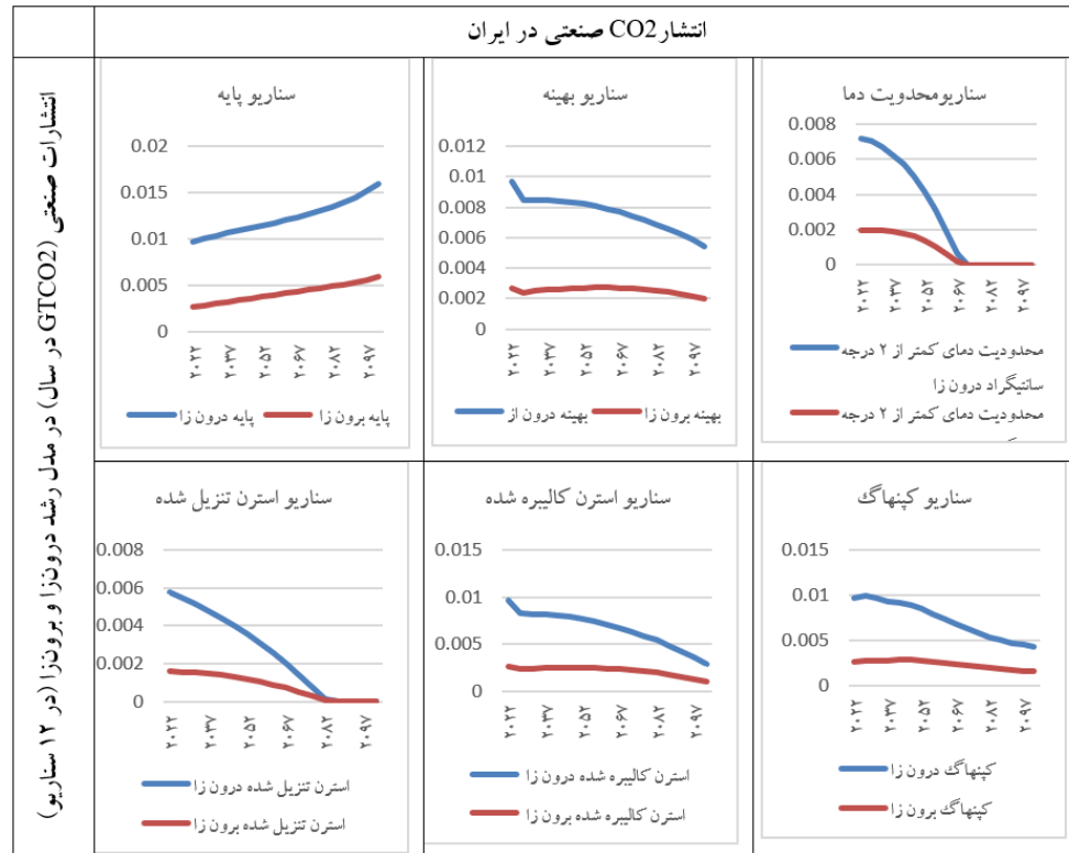
شکل (۲-الف) - انتشار پیش‌بینی شده CO2 ایران طی دوره ۲۰۲۲-۲۱۰۲ (منبع یافته‌های تحقیق)
